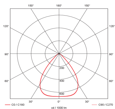
EXAIL 2122/P_T/ (105W - 12802LM) (90°X 90°)
